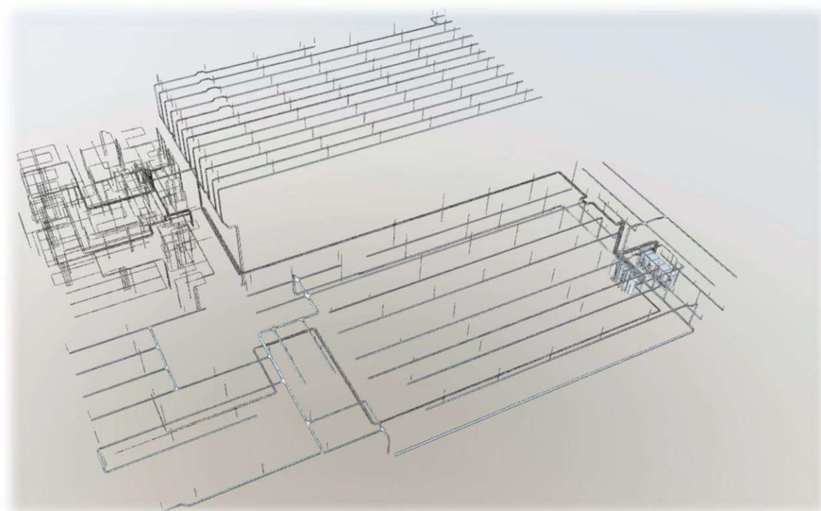
Рисунок А.19 – Подсистема «Система электроснабжения общего назначения» системы «Система электроэнергетики»
