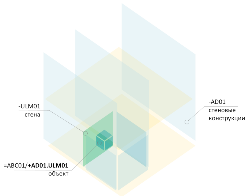
Рисунок 4.3.4.1.1 – Схематичное отображение аспекта местоположения (точка установки) для объекта с кодом «ABC01»
