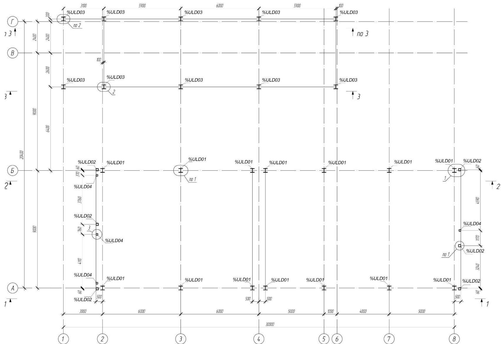
Рисунок Б.5.2 – Обозначение элементов несущего каркаса ЛЮС на разрезе
